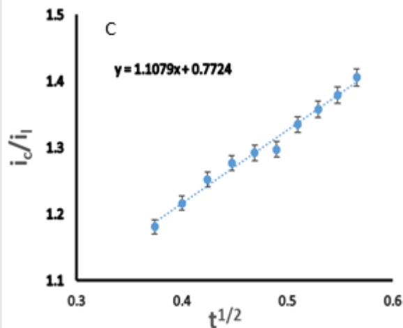
شکل ۷- (A) کروئوامپروگرام پله‌ی دوگانه الکتروود اصلاح‌شده در محلول ۰٫۱ مولار سود با غلظت‌های مختلف متانول (a): ۰٫۴، (b): ۰٫۱، (c): ۰٫۲، (d): ۰٫۴ مولار، پله‌های پتانسیل به ترتیب ۰٫۷ و ۰ ولت. (B) نمودار متانول I به S^{-1} حاصل از داده‌های کروئوامپرومتری در غلظت، ۰٫۴ مولار متانول، (C) ارتباط i_c/i_a برحسب t^{1/2} به دست آمده از داده‌های کروئوامپروگرام در بازه‌ی زمانی ۰٫۱۴ تا ۰٫۳۲ ثانیه
