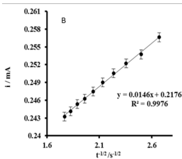
شکل ۷- (A) کروئوامپروگرام پله‌ی دوگانه الکتروود اصلاح‌شده در محلول ۰٫۱ مولار سود با غلظت‌های مختلف متانول (a): ۰٫۴، (b): ۰٫۱، (c): ۰٫۲، (d): ۰٫۴ مولار، پله‌های پتانسیل به ترتیب ۰٫۷ و ۰ ولت. (B) نمودار متانول I به S^{-1} حاصل از داده‌های کروئوامپرومتری در غلظت، ۰٫۴ مولار متانول، (C) ارتباط i_c/i_a برحسب t^{1/2} به دست آمده از داده‌های کروئوامپروگرام در بازه‌ی زمانی ۰٫۱۴ تا ۰٫۳۲ ثانیه
