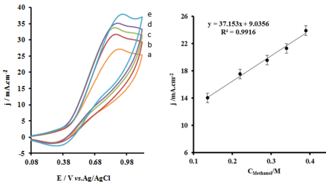
شکل ۵- ولتاموگرام چرخه‌ای حاصل از افزایش غلظت متانول در محلول ۰,۱ مولار سود، شامل غلظت‌هایی از ۰,۱۳، ۰,۲۲، ۰,۲۹، ۰,۳۴، ۰,۳۹، ۰,۴۴ مولار متانول بر روی الکتروود اصلاح شده با فیلمی از نانولوله‌های کربن، پلیمر و نانوذرات مس اکسید در شرایط بهینه آماده‌سازی الکتروود
