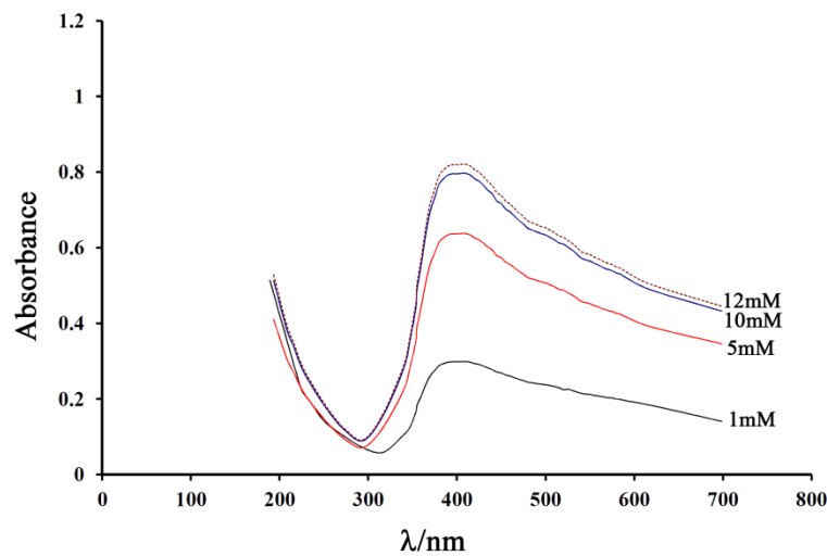
شکل ۲: طیف جذبی نانوذرات سنتزی در شرایط دمایی ۳۵ دجه سانتی گراد، و \text{pH}=1.0/0.5 و پس از ۲۴ ساعت در حضور غلظت‌های مختلف اولیه از نیترات نقره
