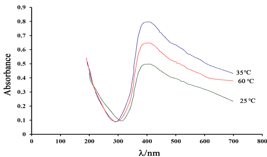
شکل ۴: طیف جذب نانوذرات سنتزی در شرایط \text{pH}=10.5 و پس از طی زمان ۲۴/۰ ساعت در حضور ۱۰/۰ میلی مولار نیترات نقره اولیه در دماهای مختلف سنتز
