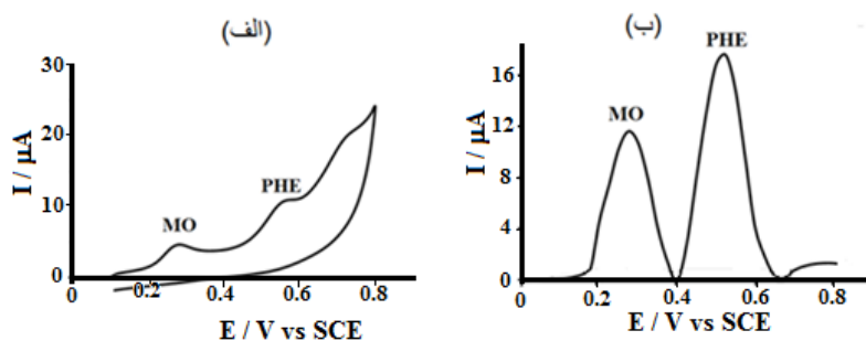
شکل ۱۲. (الف) ولتاگرام چرخه‌ای دو ترکیب مورفین و فنیل‌افرین بر روی الکترود IL/MWCNT/CCE در غلظت ۳۰ میکرومولار از دو ترکیب در محلول بافر فسفات ۰/۱M (pH=۸) و با سرعت روبش 50 \text{ mV s}^{-1} و (ب) پالس ولتاموگرام تفاضلی مخلوطی از دو ترکیب مورفین و فنیل‌افرین بر روی الکترود IL/MWCNT/CCE در غلظت ۳۰ میکرومولار از دو ترکیب در شرایط بهینه: پهنای پالس ۵۰ ms، پله پتانسیل ۵ mV، بافر فسفات ۰/۱ M (pH=۸).
